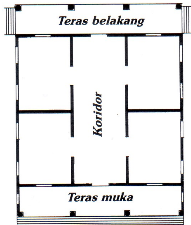
Gb.5C Typical denah rumah gaya " Indische Empire ", dengan ciri khas yaitu teras depan dan belakang sebagai bagian penting dari denahnya.
