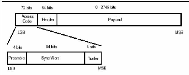
Gambar 9. Struktur Frame Data Bluetooth
