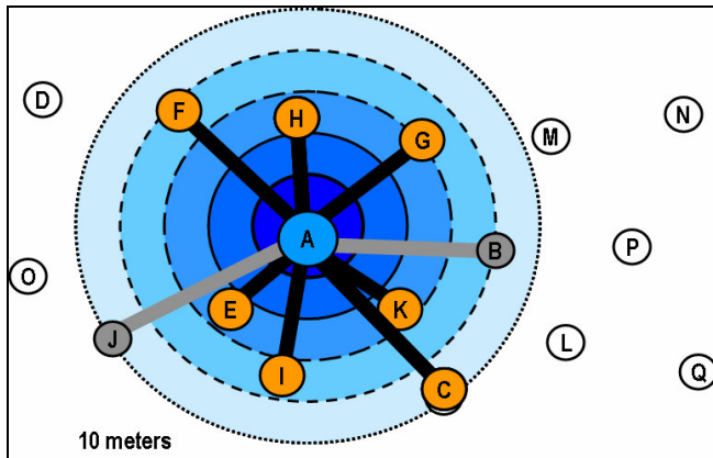
Gambar 6. Proses Mengembangkan Piconet
