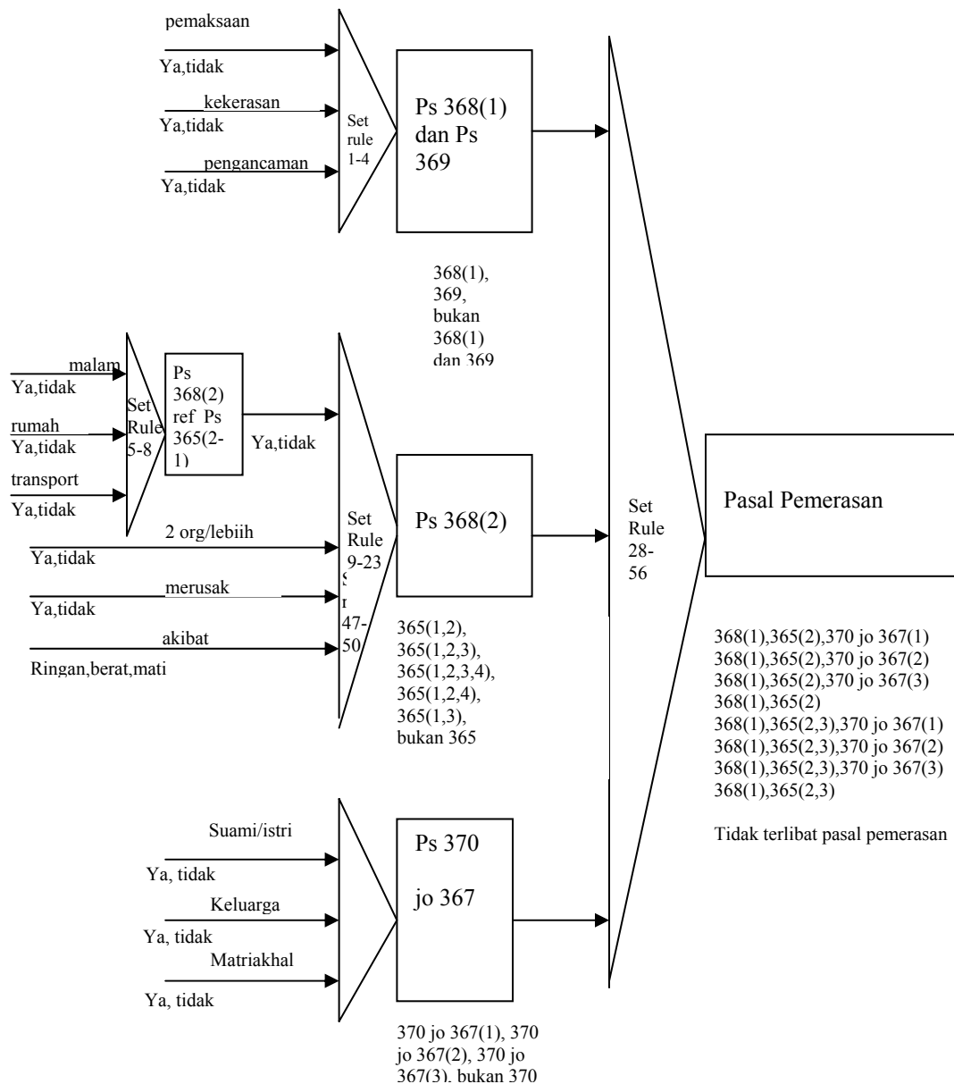
Gambar 7. Dependency Diagram Pasal-pasal Pemerasan dan Pengancaman
