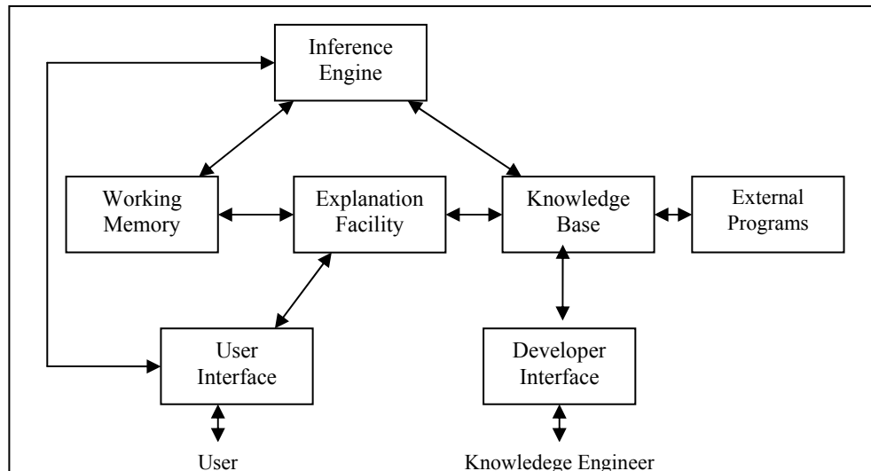
Gambar 1. Arsitektur Sistem Pakar
